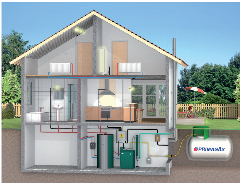
Elektrische und heizungstechnische Einbindung im Ein- und Mehrfamilienhaus mit dem Dachs SE
